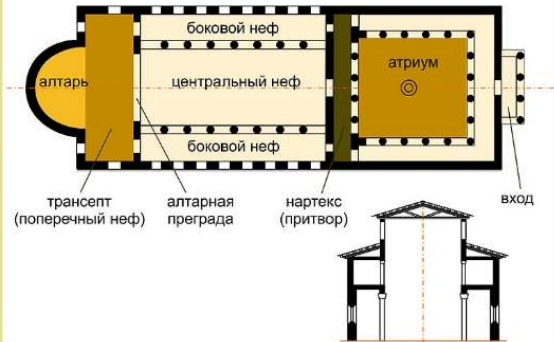
План и конструкция христианской базилики
